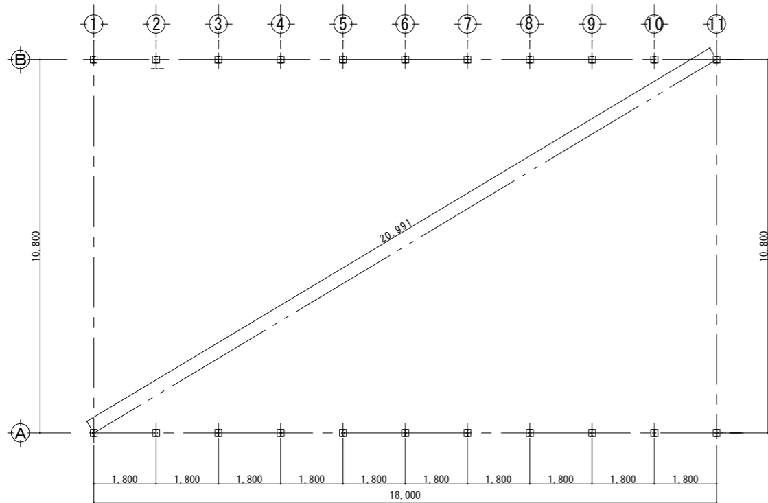
平面図・基礎伏図
