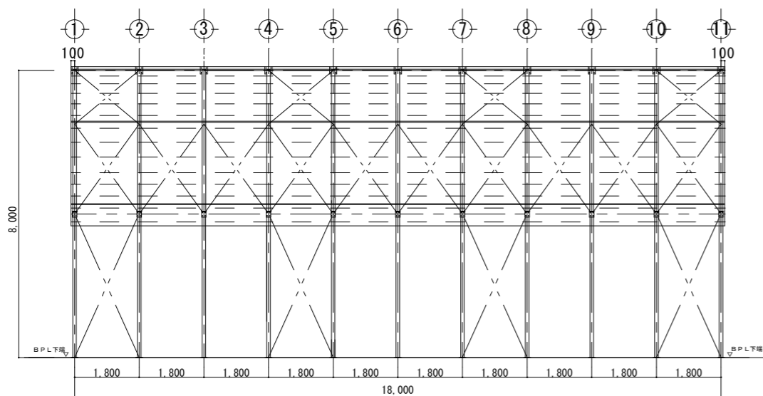
A・B通り軸組図
