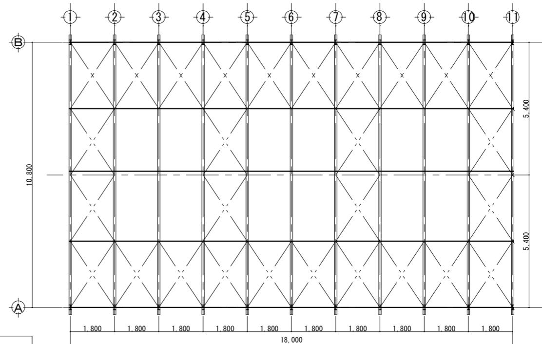
小屋伏図
